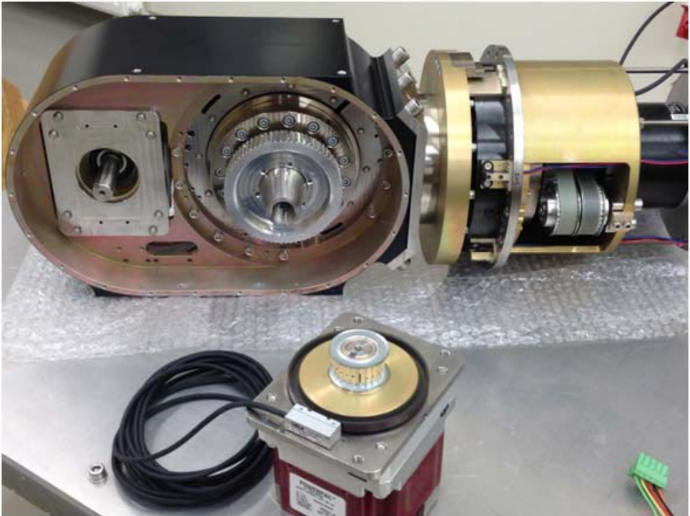
рис. 3. Элементы привода новой монтировки. rys. 3. Elementy napędu nowego montażu
