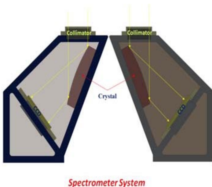
рис. 4. Детали конструкции одного из каналов системы SA и схема взаимного размещения кристаллов в блоке Спектрального атласа (SA)
