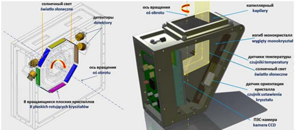
рис. 2. Слева: схема быстро вращающегося спектрометра RDS. Справа: схема поляриметра B-POL rys. 2. Po lewej: schemat funkcjonalny szybko rotującego spektrometru RDS. Po prawej: schemat polarymetru B-POL
