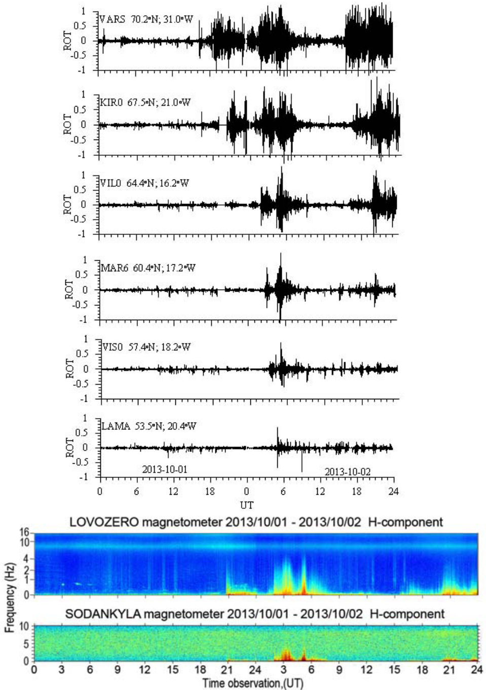
рис. 5. Широконое проявление TEC флуктуаций для 1 и 2 октября 2013 года и кеограммы для станций Ловозеро и Соданкула
