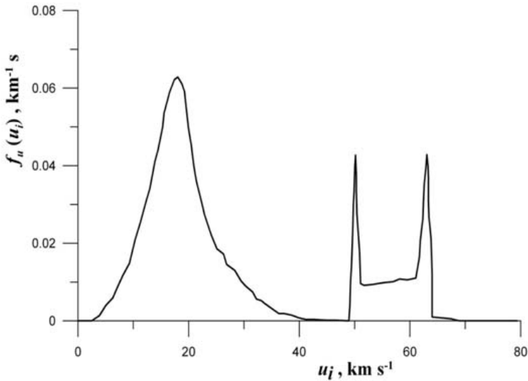
рис. 6. Функция распределения метеороидов, ударяющихся о поверхность Луны, по скоростям rys. 6. Funkcja rozkładu meteorytów uderzających o powierzchni Księżyca w zależności od prędkości.
