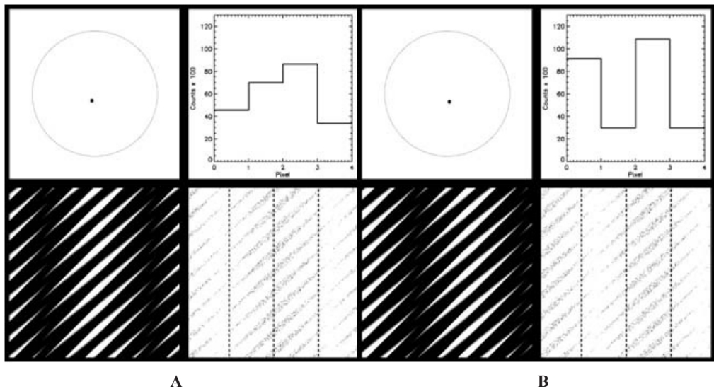
рис. 2. Результаты трассировки идеальных решеток для двух положений источника излучения на солнечном диске (А и В). Расстояние между положениями источника составляет \sim 1,5' . Левая верхняя панель: положение источника на диске Солнца. Правая верхняя панель: количество отсчетов на каждом из четырех пикселей детектора. Левая нижняя панель – картина Муара. Правая нижняя панель – распределение попаданий фотонов на поверхность детектора при пофотонной трассировке
