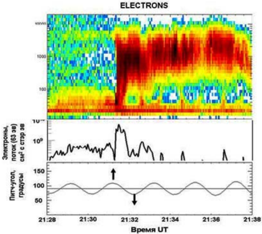
рис. 6. Верхняя панель – динамическая спектрограмма электронов; средняя панель – поток электронов с энергией 63 эВ; нижняя панель – питч-угол измеряемых электронов. Стрелками отмечено направление движение частиц.
