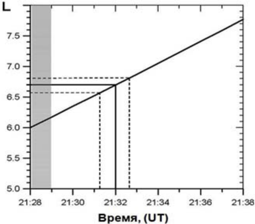
рис. 3. Изменение L -оболочки вдоль орбиты спутника ИНТЕРБОЛ-2 при пролете над нагревным стендом EISCAT в Тромсе.
