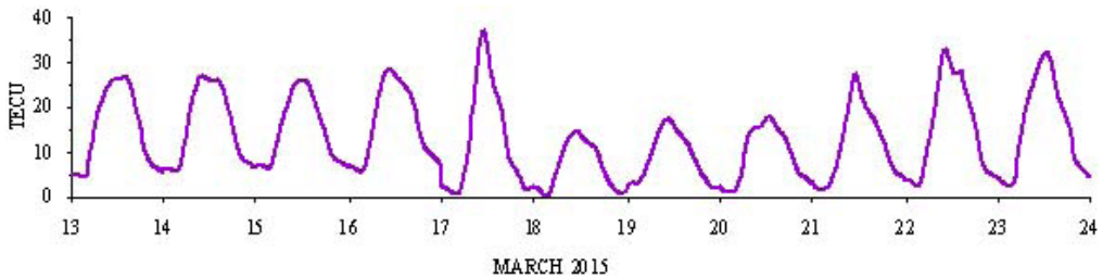
рис. 8. Суточные вариации ГЛОНАСС-TEC по станции Ламковко за период 13–23 марта 2015 года
