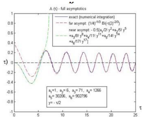
рис. 3. (а) Рельеф подынтегральной функции \tilde{R}(q)e^{-iq\tau} и контур интегрирования, проходящий через седловые точки; (б) импульсная реакция плазменного слоя с линейно растущей электронной концентрацией – точное решение и асимптотическое представление
