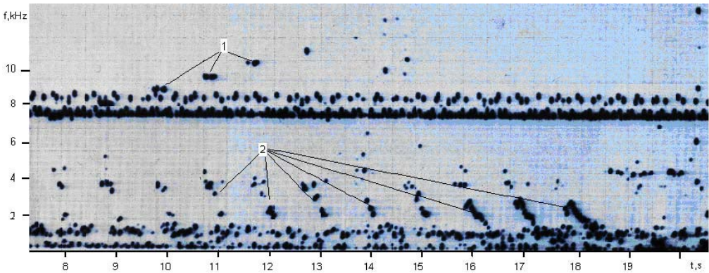
рис. 6. Спектрограмма широкополосной ОНЧ-записи сигналов (полоса 20 Гц – 20 кГц) на витке 1238 спутника «ИНТЕРКОСМОС-24» 5.01.90 г в 17 h 04' МСК. Н = 1000 км, L = 2,3. Цифрой 1 обозначены импульсы прибора ПВП с амплитудой 50 В на частотах 8,5; 9,5 и 10,5 кГц, цифрой 2 обозначены индуцированные сигналы
