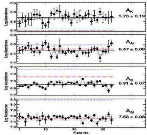
рис. 3. Усредненные по времени содержания элементов в короне по данным отдельных вспышек, а также усредненные величины содержаний элементов (черная сплошная линия) по данным всех 33 исследованных вспышек. Красные прерывистые линии соответствуют величинам «фотосферных» содержаний элементов из работы [Asplund et al., 2009] для Si, S, K, а для Ar из работы [Lodders et al., 2008]. Голубые пунктирные линии соответствуют величинам «корональных» содержаний из работы [Feldman, 1992] для Si, S, Ar, а для K из базы CHIANTI.
