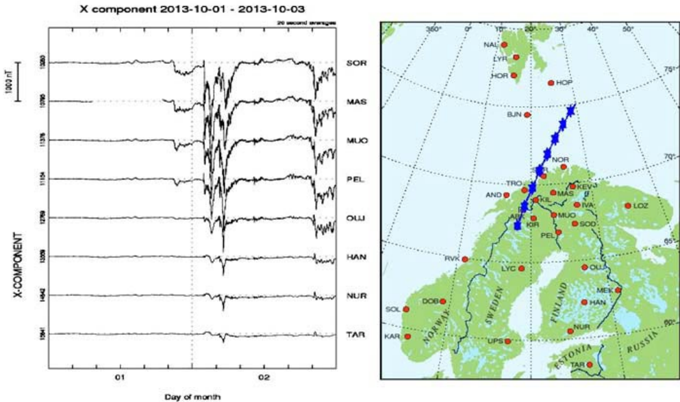
рис. 2. Вариации геомагнитного поля (X-компонента) (слева) на станциях, разнесённых по широте скандинавской сети и карта расположения магнитометров (справа)
