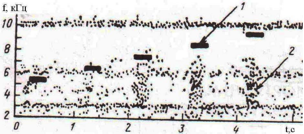
рис. 2. Спектрограмма записи ОНЧ-сигналов в полосе 2–10 кГц при работе ПВП на витке 941 спутника «ИНТЕРКОСМОС-24»
