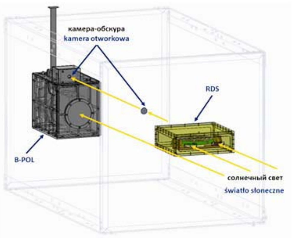
рис. 1. Распределение модулей прибора СОЛЬПЕКС внутри аппаратуры КОРТЕС rys. 1. Rozmieszczenie bloków pomiarowych instrumentu SOLPEX wewnątrz platformy KORTES
