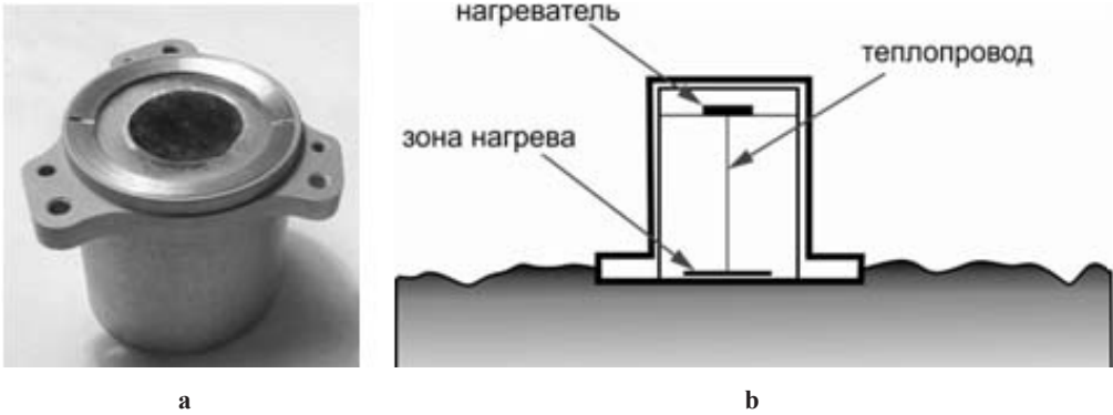
рис. 1. Внешний вид (а) и принципиальная схема (б) поверхностного термодатчика ПТД rys. 1. Zdjęcie (a) i diagram schematyczny (b) STS
