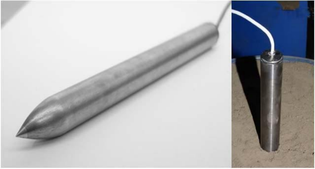
Рис. 6. Пенетратор EMOLE (слева), этот пенетратор во время теста (справа)
