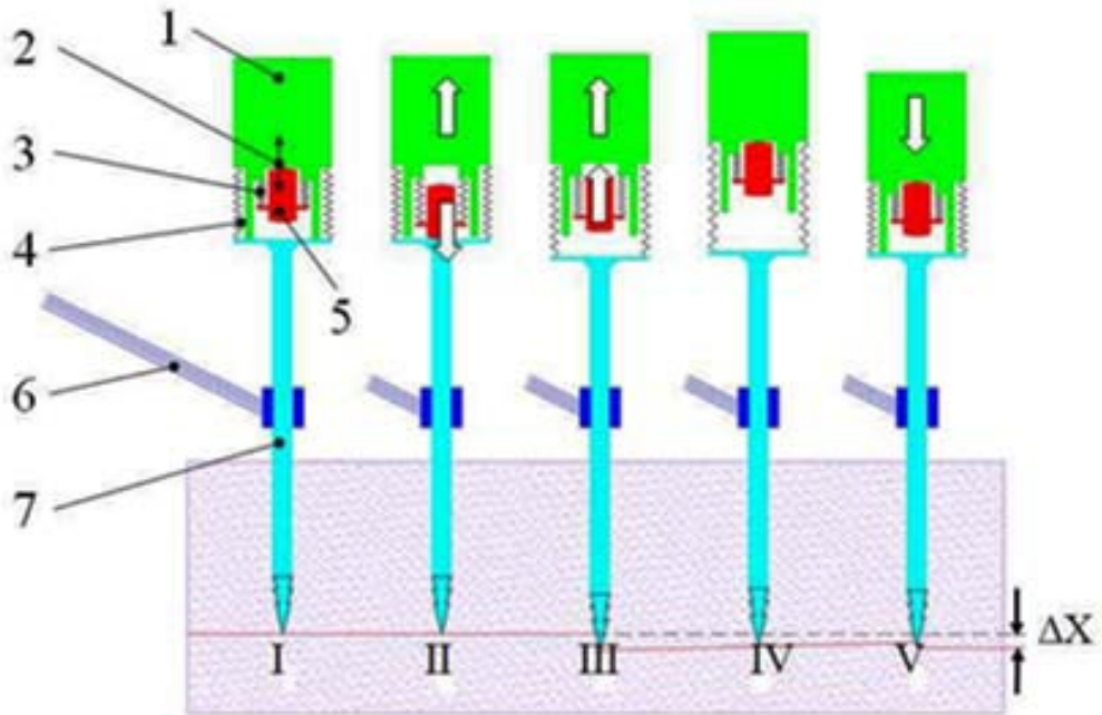
рис. 4. Принцип работы пенетратора MUPUS (основные части: 1 – контрмасса; 2 – место генерации ударной силы; 3 и 4 – пружинные подвески; 5 – ударник; 6 – рычаг манипулятора (1 м), заканчивающийся направляющим зажимом (0-1N); 7 – стержень) rys. 4. Zasada działania penetratora MUPUS (główne części: 1 – przeciwmasa; 2 – miejsce generowania siły uderzenia; 3 i 4 – zawieszenie sprężyste; 5 – młotek; 6 – ramię manipulatora (1 m) zakończone zaciskiem ołowiowym (0-1N); 7 – pręt).
