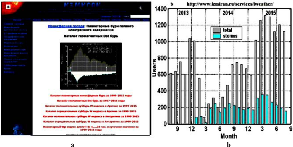
рис. 1. (а) Страница «Бури» на сайте «Ионосферная погода» ИЗМИРАН, включая график геомагнитно-ионосферной супер бури 17-21 марта 2015 года; (б) Число пользователей сайта «Ионосферная погода» ИЗМИРАН и «Бури» за каждый месяц с августа 2013 по август 2015 года.
