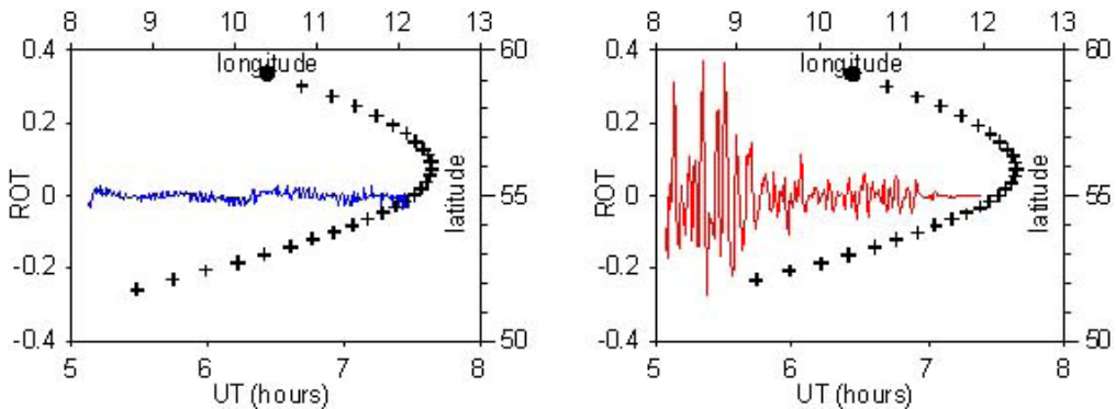
рис. 4. ТЕС флуктуации на станции Ламковко для спутника № 14 для спокойного (слева) и возмущённого (справа) дней rys. 4. Fluktuacje TEC nad stacją Lamkówko dla satelity nr 14 dla spokojnego (lewa strona) i zaburzonego (prawa strona) dnia
