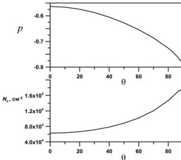
рис. 2. Величины p и N_e в зависимости от угла \theta для участков лунного реголита rys. 2. wielkości p i N_e w zależności od kąta \theta dla fragmentów księżycowego
