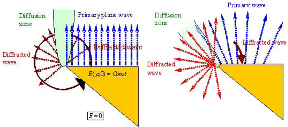
рис. 1. Излучение плоской волны, колеблющейся гранью клина, и более общее краевое условие rys. 1. Promieniowanie fali płaskiej od oscylującej krawędzi klina i przypadek uogólnionych warunków brzegowych
