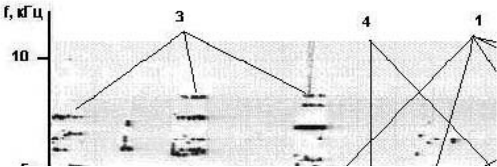
рис. 5. Спектрограмма ОНЧ-сигнала в полосе 0–10кГц. Начало цикла с амплитудой 100 В. Явление затяжки импульса выражено почти на всех частотах. Сигналы с падающим спектром имеют малую интенсивность. Обозначения те же, что и на рис. 3. Орбитальные данные в пределах погрешности совпадают с данными того же рисунка
