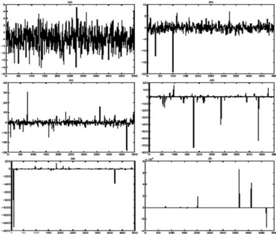
рис. 5. Примеры случайных последовательностей с параметром \alpha = 2,0; 1,95; 1,5; 0,85; 0,45 rys. 5. Przykłady sekwencji losowych z parametrem \alpha = 2,0; 1,95; 1,5; 0,85; 0,45
