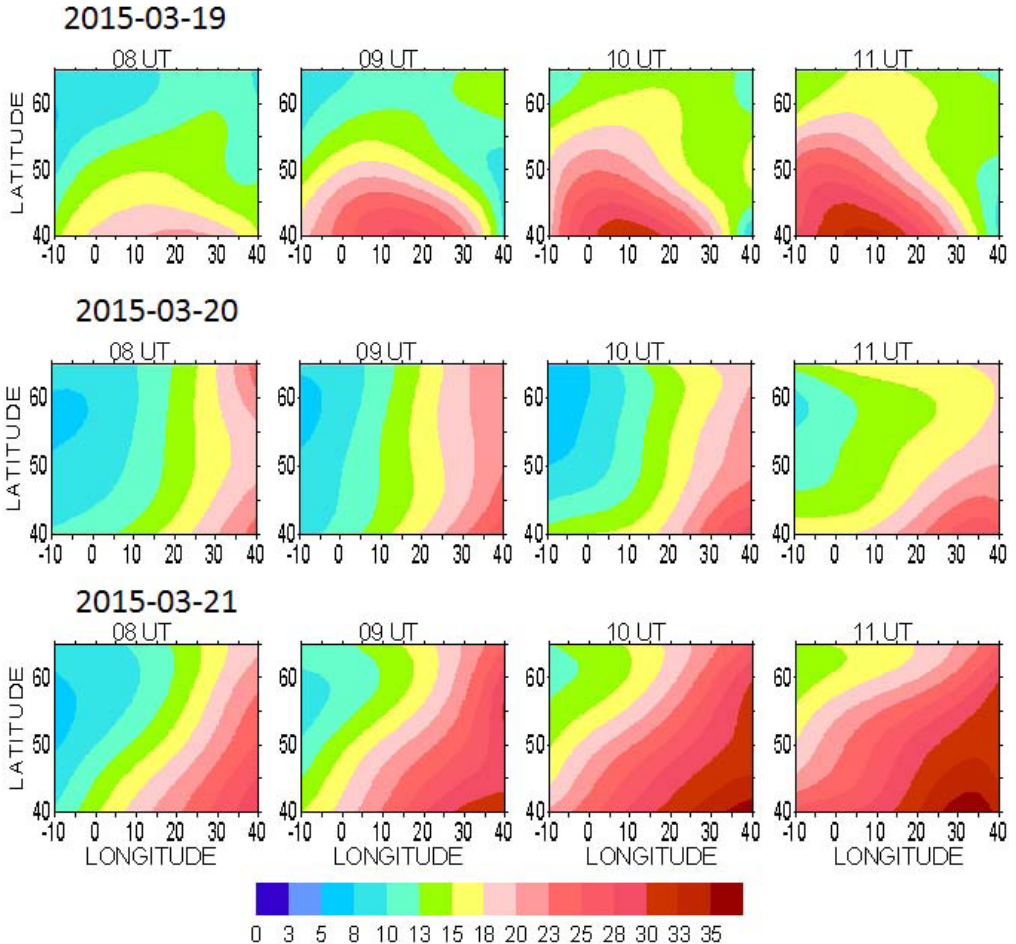
рис. 9. GLONASS-TEC карты над Европой 19, 20 и 21 марта 2015 г.
