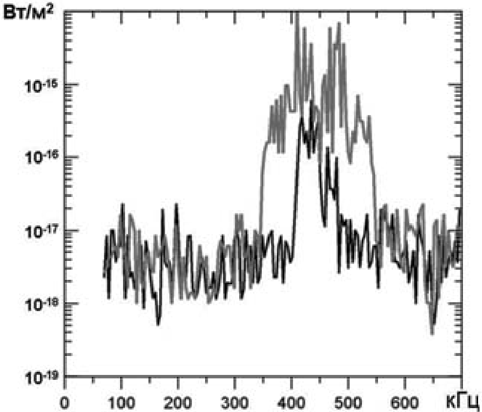
рис. 5. Спектры АКР, измеренные в 21:28:41 UT – до входа спутника в сопряженную силовую трубку (серая кривая) и в 21:31:55 UT – внутри силовой трубки (черная кривая).
