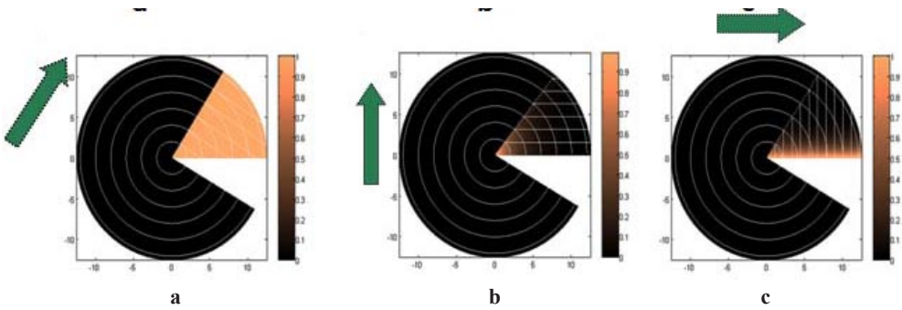
рис. 2. Излучение волн источником, распределенным вдоль грани клина: область существования и картина волновых фронтов для однородной (а), неоднородной (b) и поверхностной (c) плоской волны
