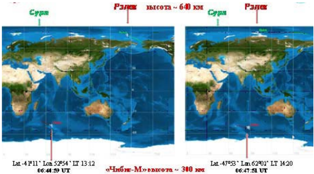
рис. 16. Пространственное распределение в синхронном эксперименте «Вернов» – «Чибис-М» – стэнд Сура
