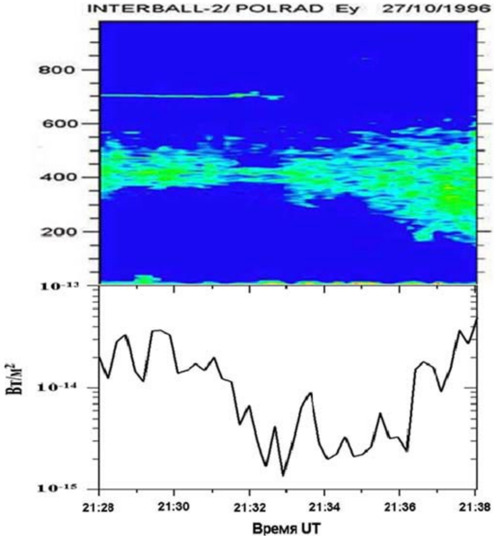
рис. 4. Динамическая спектрограмма АКР по измерениям со спутника ИНТЕРБОЛ-2 (верхняя панель). Интегральная мощность излучения АКР (нижняя панель).
