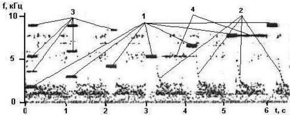
рис. 3. Спектрограмма ОНЧ-сигнала в полосе 0–10 кГц при работе ПВП с амплитудой 50 В на витке 1238 спутника «ИНТЕРКОСМОС-24». Начало цикла в 17 h 02'20'' МСК ( t = 0 с).
