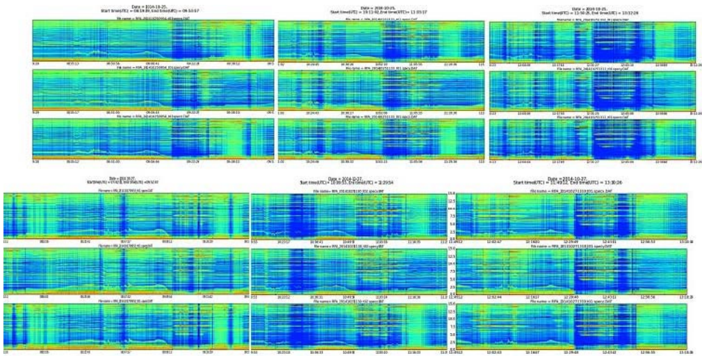
рис. 14. Пример данных РЧА за 25 и 27 октября 2014 г. rys. 14. Przykładdane zarejestrowane RFA 25 i 27 października 2014 r.
