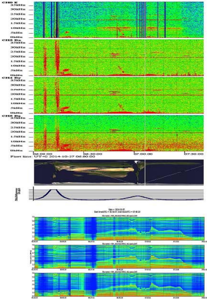
рис. 17. Синхронные данные НЧА и РЧА 27.10.2014 года 06:00:00–07:42:00 UT. Первая (верхняя) панель – электрическая компонента НЧА в диапазоне <40 \text{ кГц} ; 2–4-я панели – три ортогональные магнитные компоненты НЧА в диапазоне <40 \text{ кГц} ; 5-я панель – проекция орбиты спутника «Вернов» на земную поверхность; 6-я панель – значения L-параметра; 7–9 панели – три ортогональные электрические компоненты РЧА в диапазоне <15 \text{ МГц} rys. 17. Dane synchroniczne NChA i RFA 27.10.2014 06:00:00–07:42:00 UT. Pierwszy (górný) panel – elektryczny komponent... w zakresie <40 \text{ kHz} ; 2–4 panele – trzy ortonormalne składowe magnetyczne... w zakresie <40 \text{ kHz} ; 5 panel – projekcja orbity sztucznego satelity „Vernov” na ziemską powierzchnię; 8 panel – wartość L-parametru; panele 9–11 – trzy prostokątne elektryczne komponenty RFA w zakresie <15 \text{ MHz}
