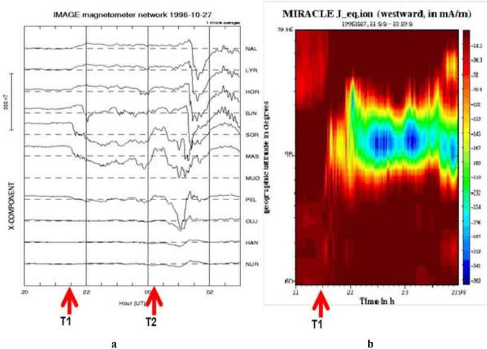
рис. 2. (а) Вариации геомагнитного поля на сети наземных станций IMAGE 27 октября 1996 года, расположенных вблизи нагревного стенда. T1 – начало работы стенда, T2 – начало классической суббури. (б) Изменение распределения эквивалентных токов в ионосфере при работе нагревного стенда Тромсе.
