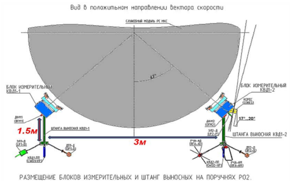
рис. 9. Схема размещения измерительных баз rys. 9. Schematy pomiarowe rozmieszczenia sensorów
