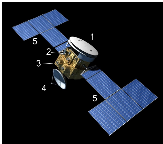
Рис. 1. Схематический вид КА Интергелиозонд и его основные системы: 1- защитный экран, 2 - платформа с комплексом научной аппаратуры, 3 - двигательная установка, 4-антенна, 5 - солнечные панели . Размеры КА 3.7 × 4.5 × 3.7 м.
